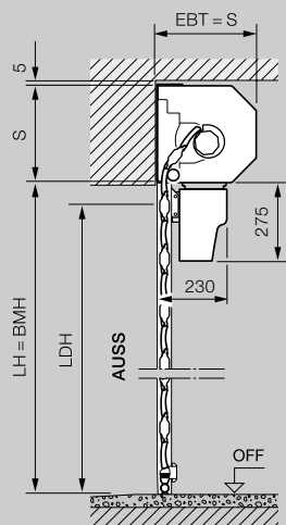
Rozsah veľkostí vnútornej a vonkajšej rolovacej brány
